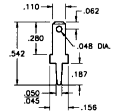
.110 TAB
