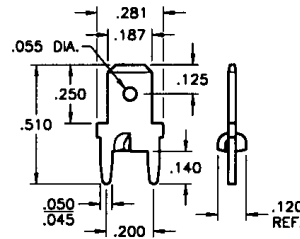
.187 TAB
